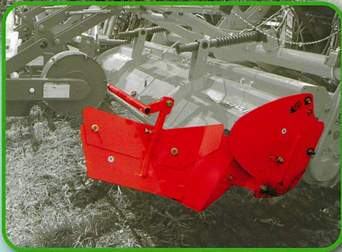
うね盛板3型
