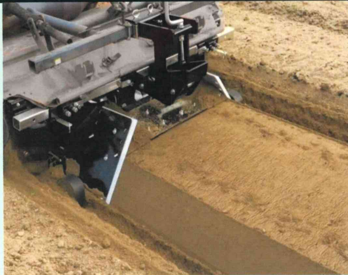
SD型での平高うねたて作業
